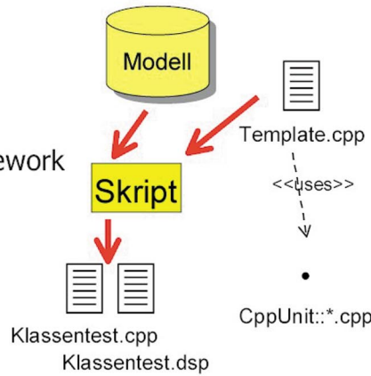
Abb. 5: Automatische Generierung von Komponenten- und Klassentests
